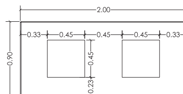
MESA VISTA INFERIOR
