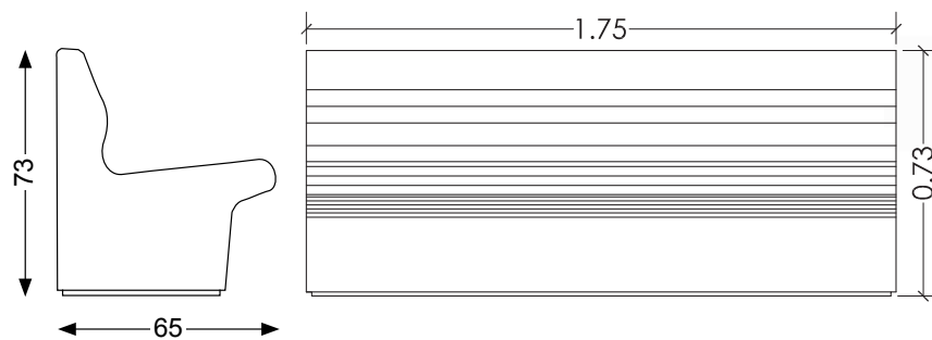
BANCO K RECTO
