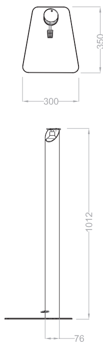
DISPENSADOR DE PEDAL
