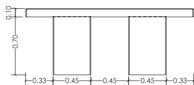
MESA ALZADO LONGITUDINAL
