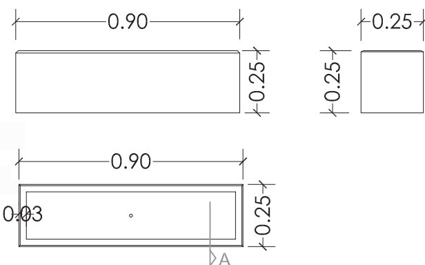
JARDINERA TRES CANTOS
