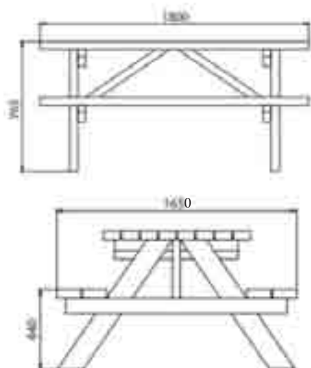
MESA PICNIC MADERA TÉCNICA
